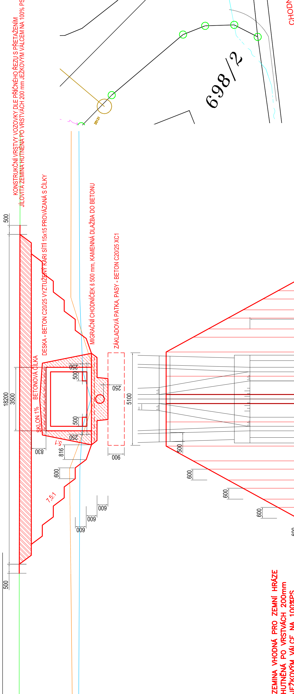
DETAIL PROVEDENÍ PŘEKOPU HRÁZE
