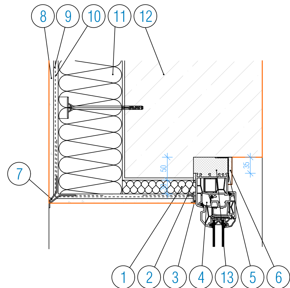
DETAIL NADPRAŽÍ OKNA :
