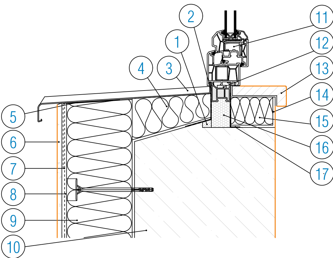
DETAIL PARAPETU OKNA :
